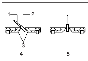
1. Пильный диск 2. Зубья диска 3. Планка для пропилов 4. Резка со скосом влево 5. Прямая рез
